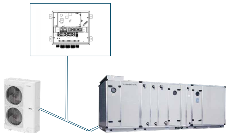
Rysunek poglądowy podłączenia zestawu AHU KIT do agregatu skraplającego przy centrali wentylacyjnej.
